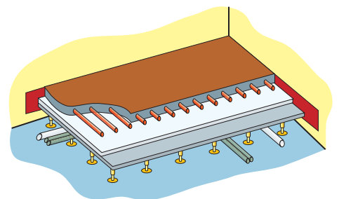
Fußbodenheizung
