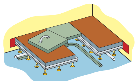
Doppelbodenkanal
