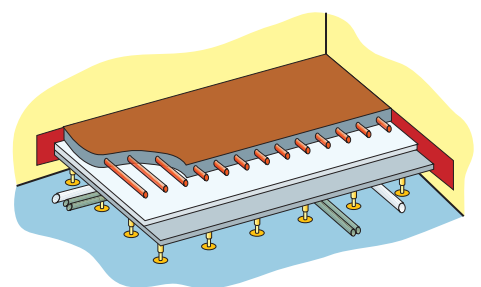
Fußbodenheizung
